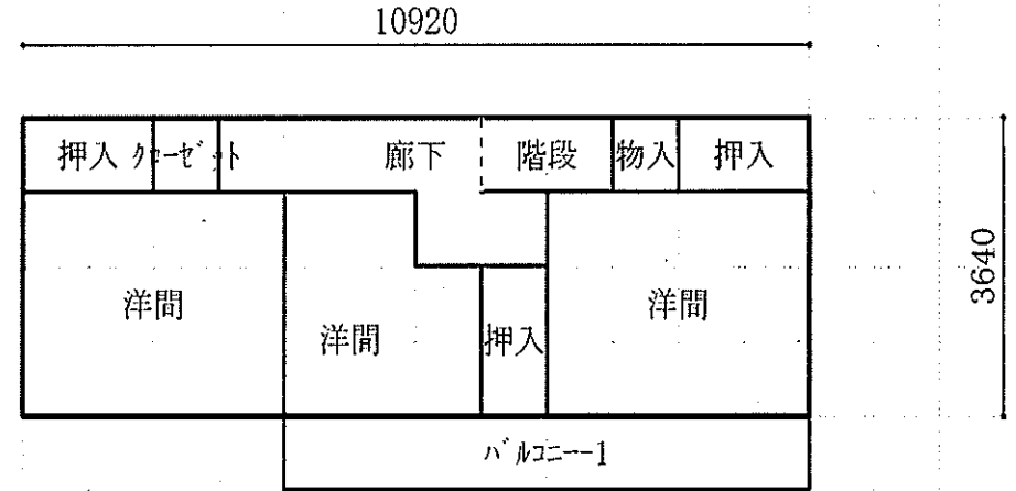
2階平面図
